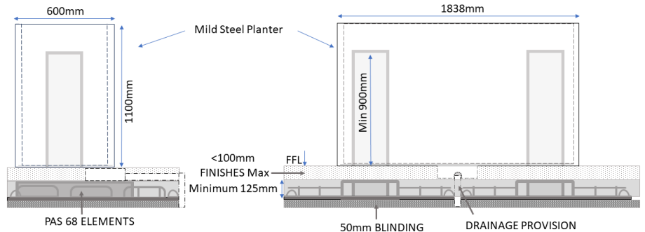
VICTORIA PAS 68 PLANTER VED 00183S USM – FOUNDATION FOOTPRINT 4540 mm (L) x 1685mm (W) x 125-225mm (D)
